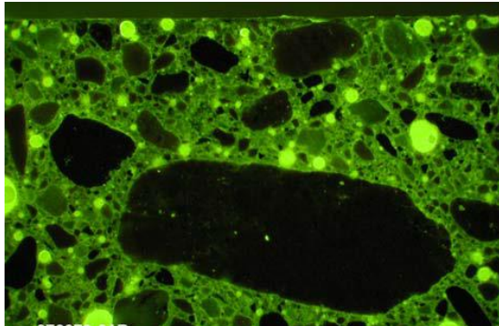
Mikroskopische Aufnahme im UV-Licht eines Betons mit künstlich eingeführten Luftporen (gelb). Die gleichmässige Verteilung, der Gehalt, der Abstand und die Grösse der Luftporen bestimmen die Wirkung als Expansionsraum für das gefrierende Porenwasser. Vergrösserung: ca. 4x, Bildbreite entspricht 2 cm
