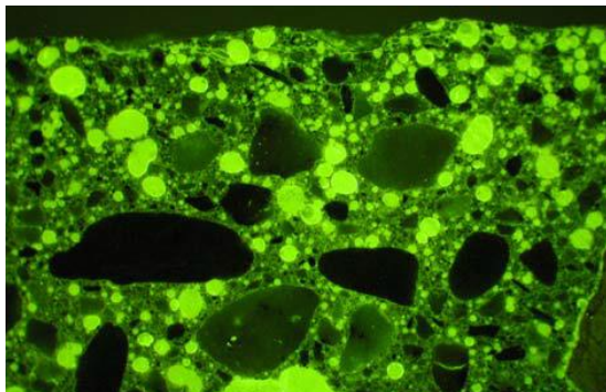
Mikroskopische Aufnahme im UV-Licht eines Betons mit künstlich eingeführten Luftporen (gelb). Zu viele Luftporen, die auch Agglomerate bilden, schwächen das Gefüge. An der Oberfläche haben sich feine Ablätterungen durch die Frostausalzeinwirkung gebildet. Vergrösserung: ca. 4x, Bildbreite entspricht 2 cm
